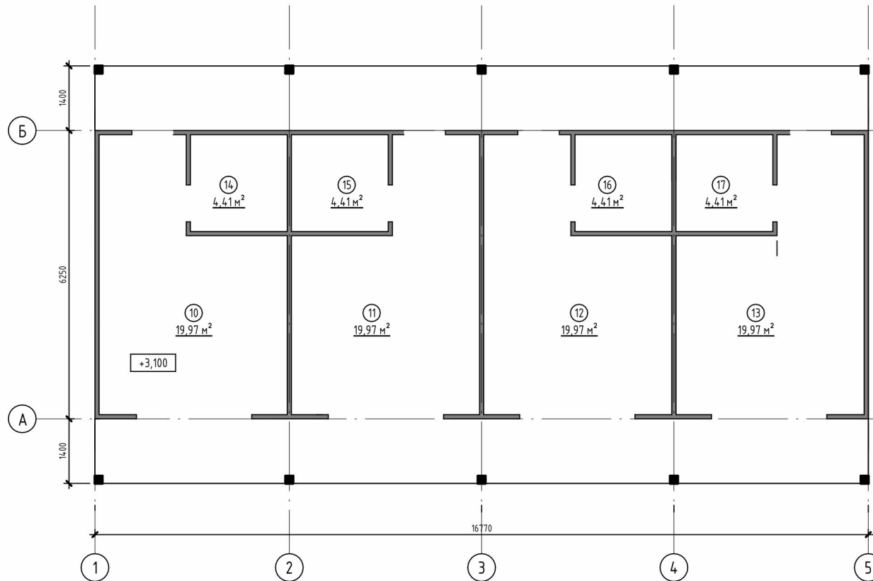
Экспликация помещений
