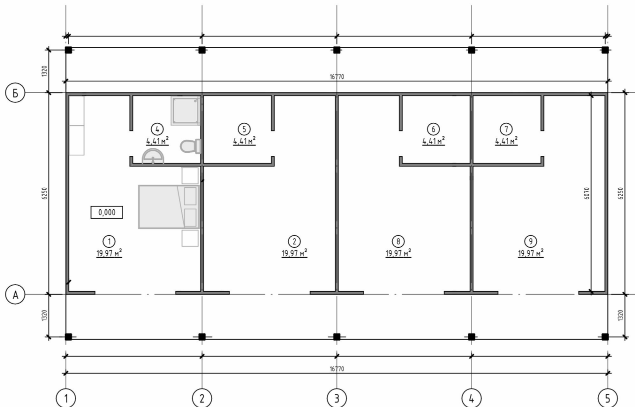
Экспликация помещений
